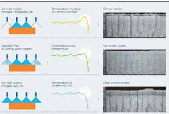
شکل ۲- اثر استفاده از نازل های آب پاش شرکت پریمتالز بر کاهش عیوب شمش ریخته‌گری مداوم.
