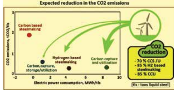
شکل ۱- پیش بینی اثرگذاری مسیرهای کاهش انتشار CO2 در صنعت آهن و فولاد
