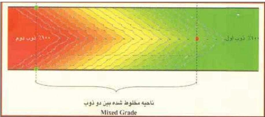
شکل ۲: الگوی اختلاط (Intermixing) در ناحیه بین دو ذوب مخلوط شده در تختال منجمد شده
