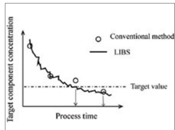
شکل ۳- مقایسه فرایند کلی کنترل غلظت کلی عناصر در مذاب با استفاده از دوروش معمولی LIBS
