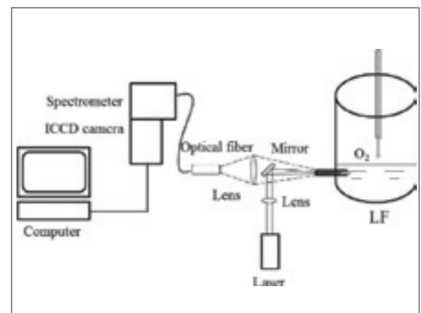
شکل ۲- کاربرد LIBS در LF
