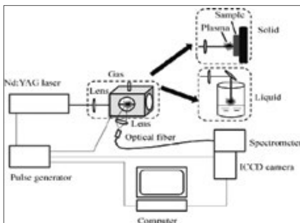
شکل ۱- آرایش هندسی LIBS
