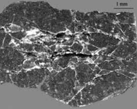
شکل ۲. تشکیل ریزترک ها در سنگ معدن پس از خردایش در HPGR.
