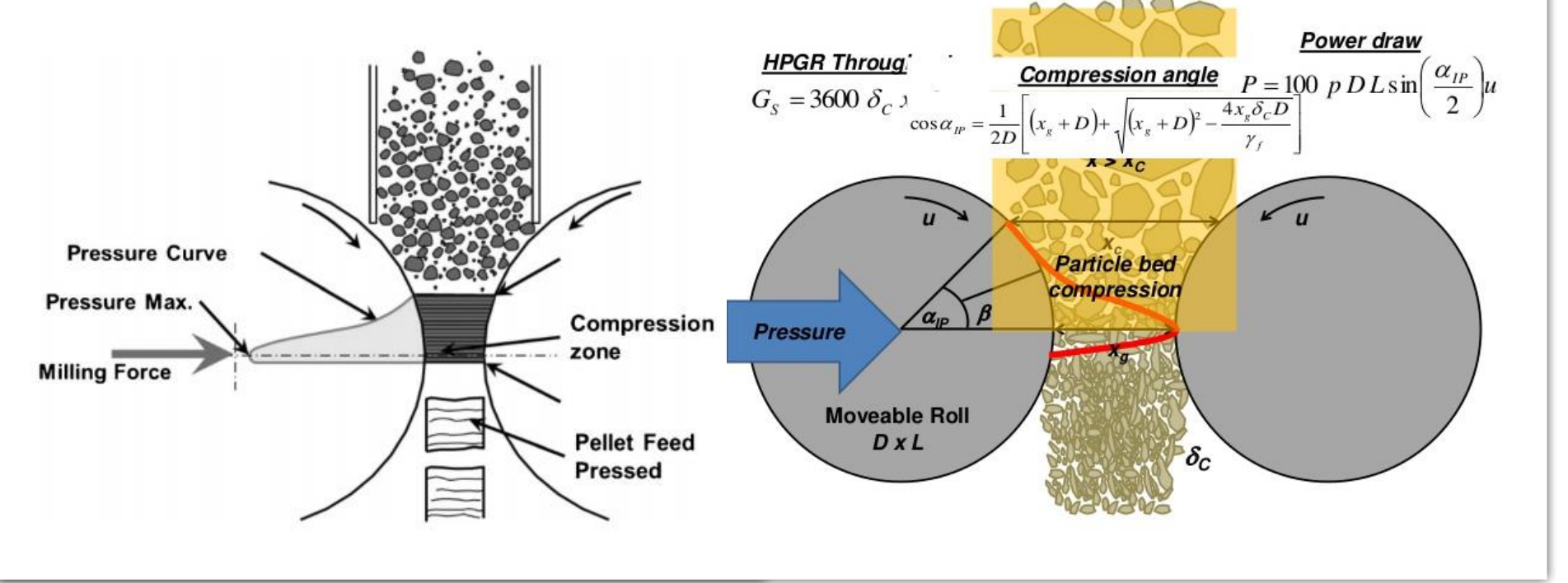
شکل ۱. نحوه توزیع نیرو در سیستم HPGR.
